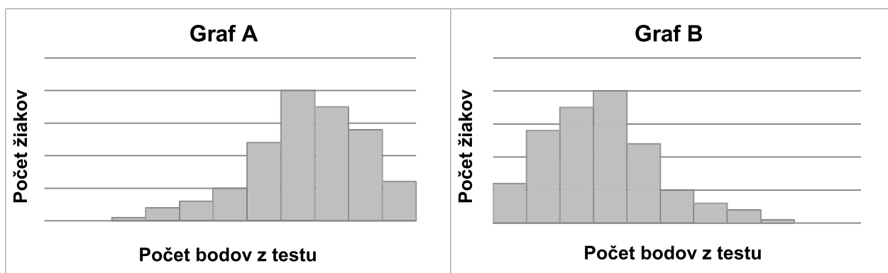
Obrázok 7. Grafy rozloženia skóre žiakov (histogramy)
