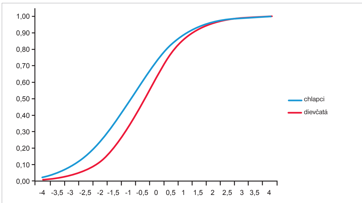
Obrázok 24. Ukážka odlišne fungujúcej úlohy a grafické zobrazenie uniformného DIF
