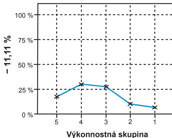
Obrázok 11. Položka so zápornou rozlišovacou schopnosťou
